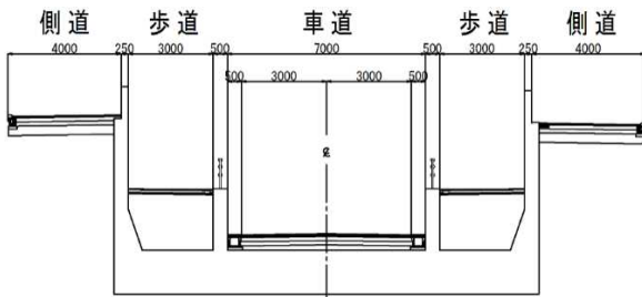
計画断面図[立体交差部]
