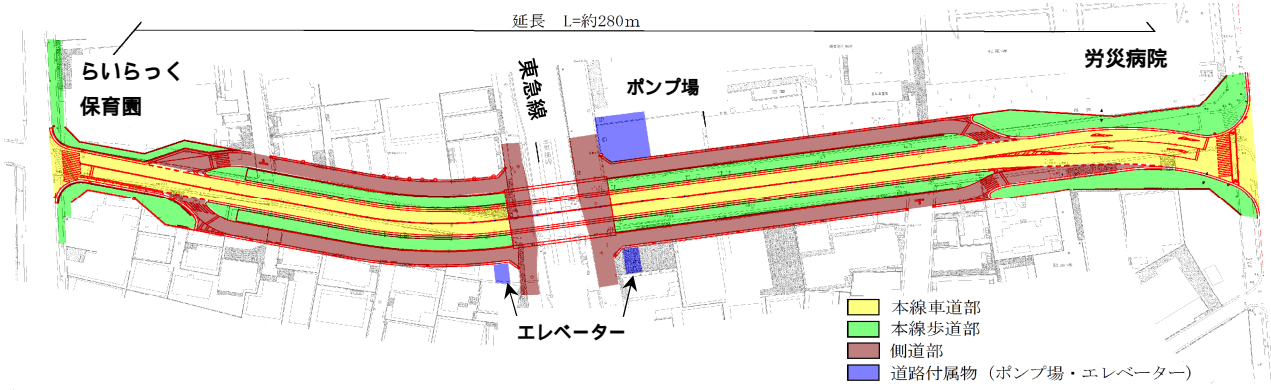
計画平面図
