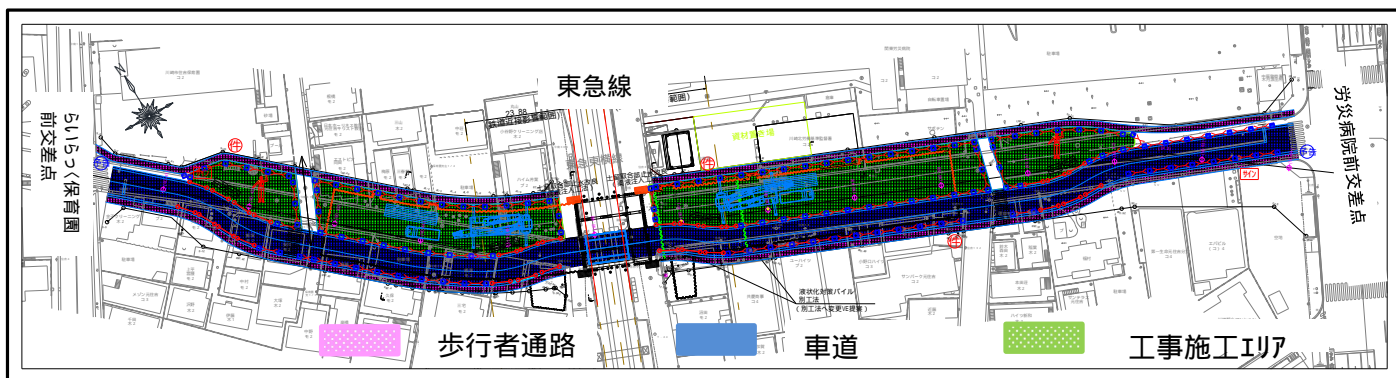
仮設道路切替後の道路形態図
