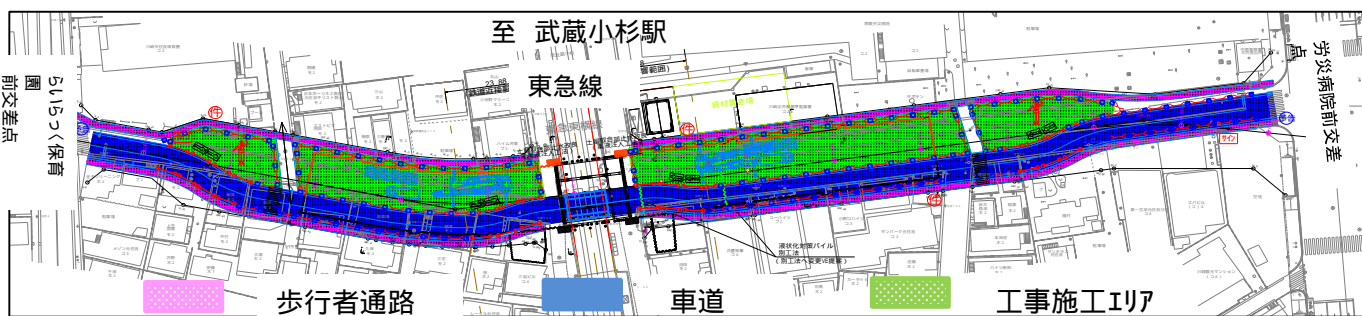
—道路形態図—
